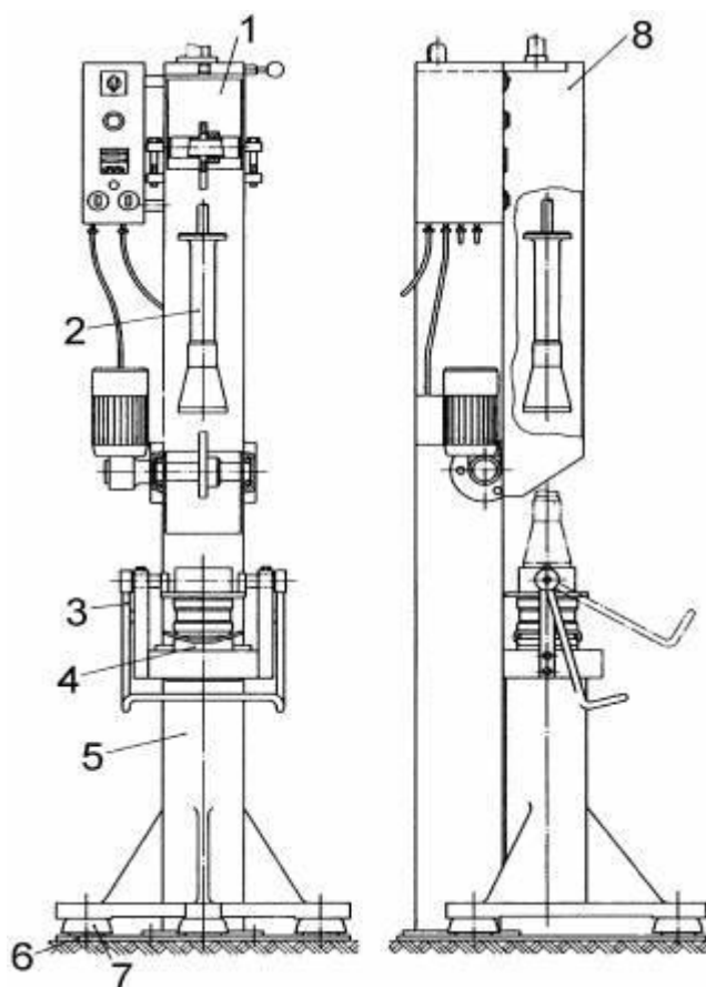
9.9-1 attēls. Trieciena blīvētāja shematiskais attēls
