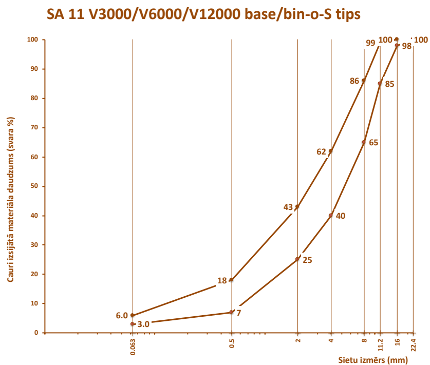
6.3-17 tabula. Prasības mīkstā asfalta SA 11 V3000/V6000/V12000 base/bin-o-S tips maisījuma granulometriskajam sastāvam
