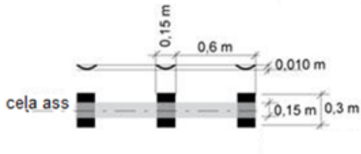
7.13-2 Attēls. Darbu izpildes tehnoloģiskā shēma
